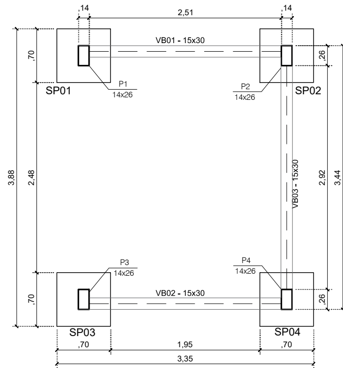
ESTRUTURA FORMA DA FUNDAÇÃO (NÍVEL -10cm) ESC: 1:50
