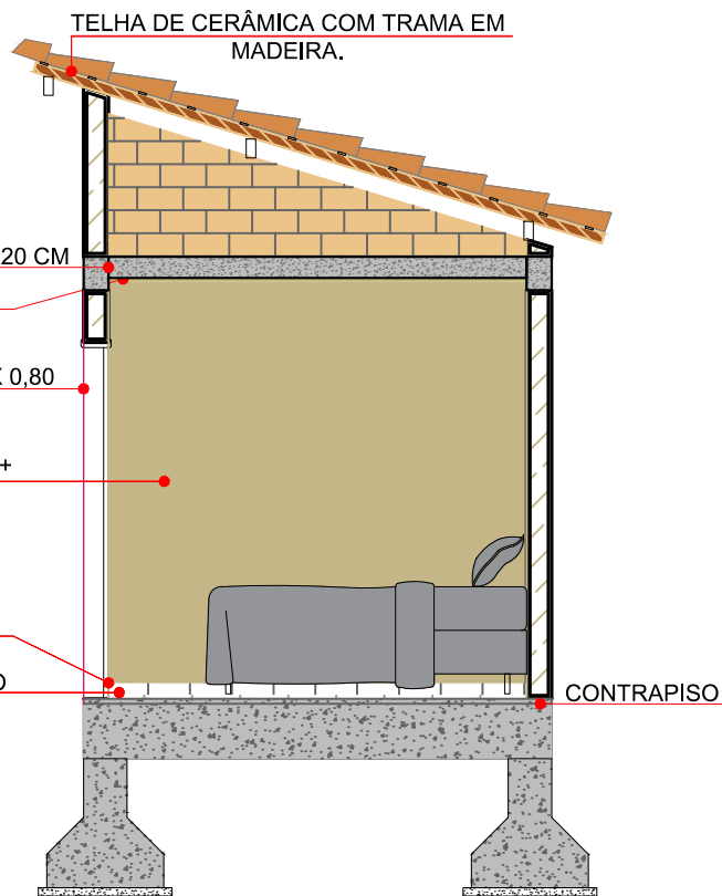
PROJETO CORTE ESC: 1:50
