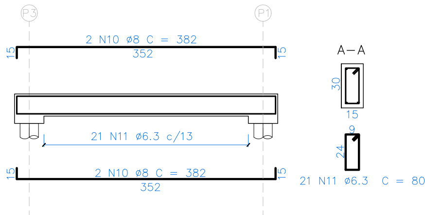
ESTRUTURA DETALHAMENTO DAS VIGAS BALDRAMES ESC: 1:50
